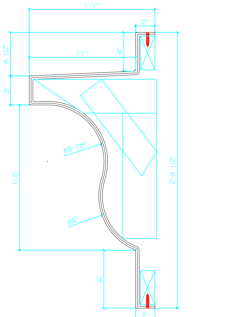
SECTION THRU CR-119X8 SCALE 1:1
